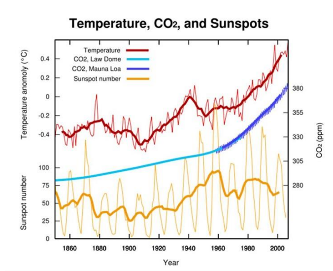
Graf 2: Vývoj koncentrací CO 2 a průměrných teplot povrchu země v letech 1850–2010.
